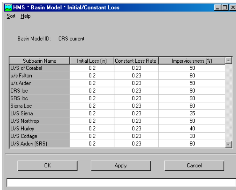
Figure 23. Alter parameter values using global editor
